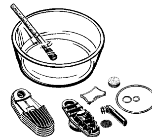
Pulizia manuale dell'Unità di Raffreddamento smontata
